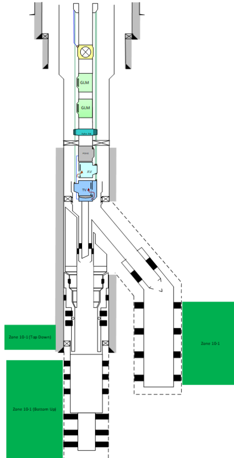
Рис.5 Схема многоствольной скважины
